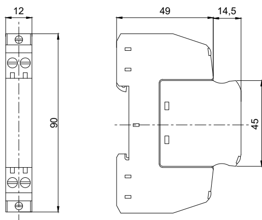
Габаритные размеры
